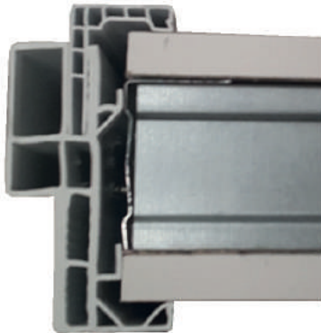
COLOCACIÓN SOBRE TABIQUE DIRECTO CARTÓN YESO PLACA SIMPLE
