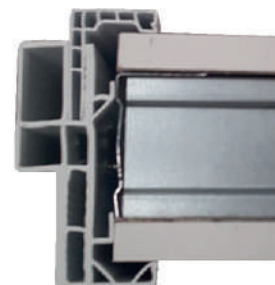
COLOCACIÓN SOBRE TABIQUE DIRECTO CARTÓN YESO PLACA SIMPLE EMBOCADURA DE REMATE SIN TAPAJUNTAS
